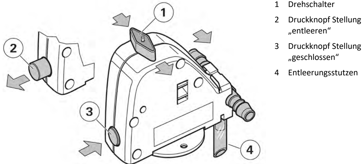
Abllassventil „FrostControl“
