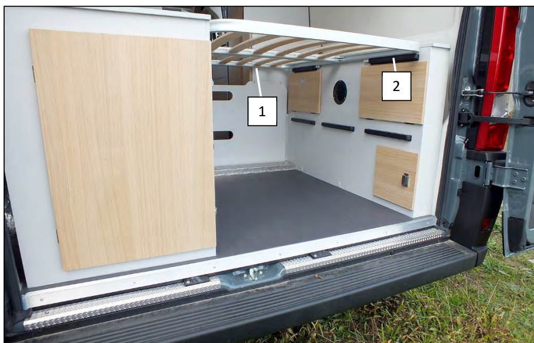
Aufgelegter Lattenrost beim Dexter 580 (Abb. beispielhaft)
